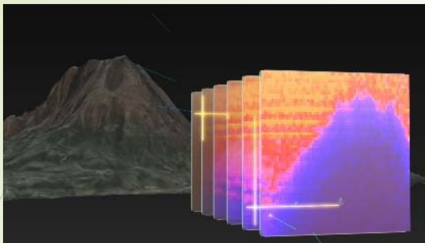
ミュオグラフィの計測原理の可視化
